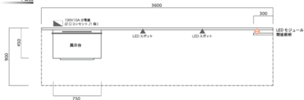
立面図
